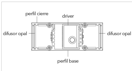
DIBUJO PERFIL
