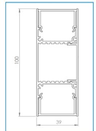
PERFIL DOBLO
